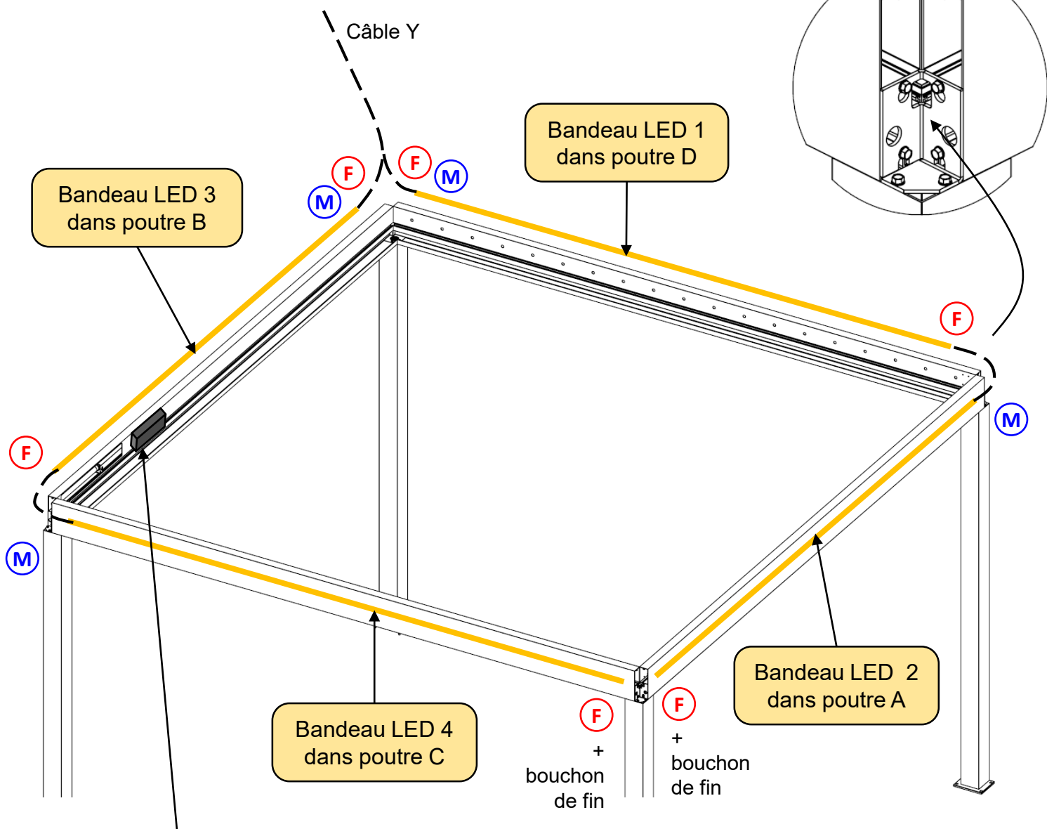
Boîtier de raccordement
