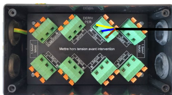
Fig. 2 Boîtier de raccordement
